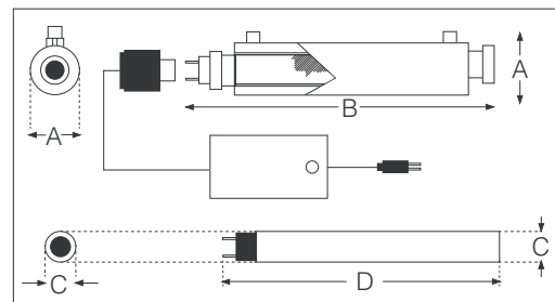
OSRAM U.V. lamp scheme
